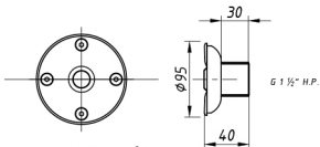
Схема установки:
